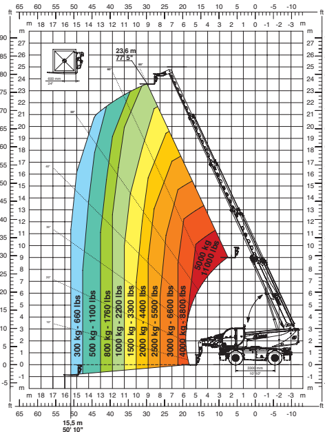
W 3,5 Argano 3,5 tonnellate
